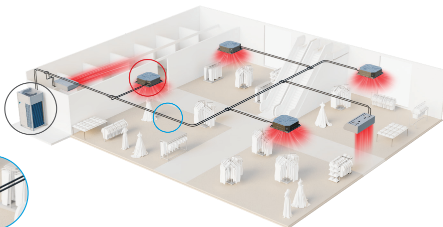
Circuito del refrigerante a 2 tubi
