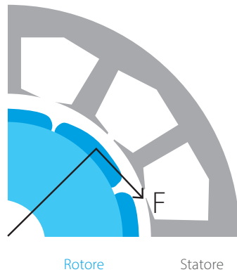
Motore convenzionale con rotore interno
