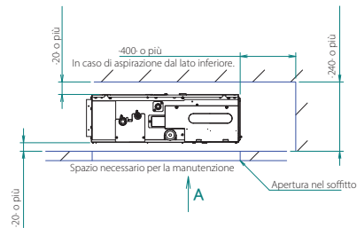
Vista A- Portello d'ispezione Apertura nel soffitto
