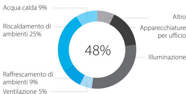
Consumi energetici medi - uffici
