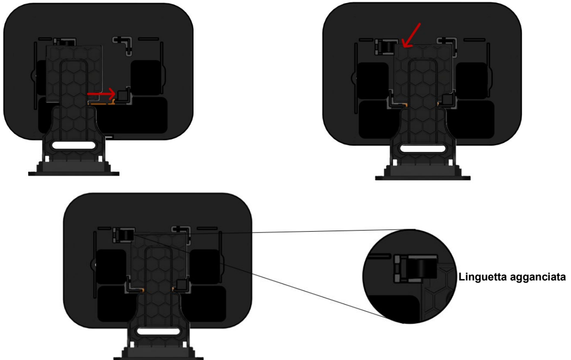
Figura 5 Aggancio piedistallo al Controller
