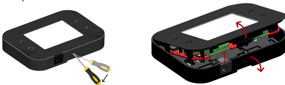
Figura 19 Apertura Controller
