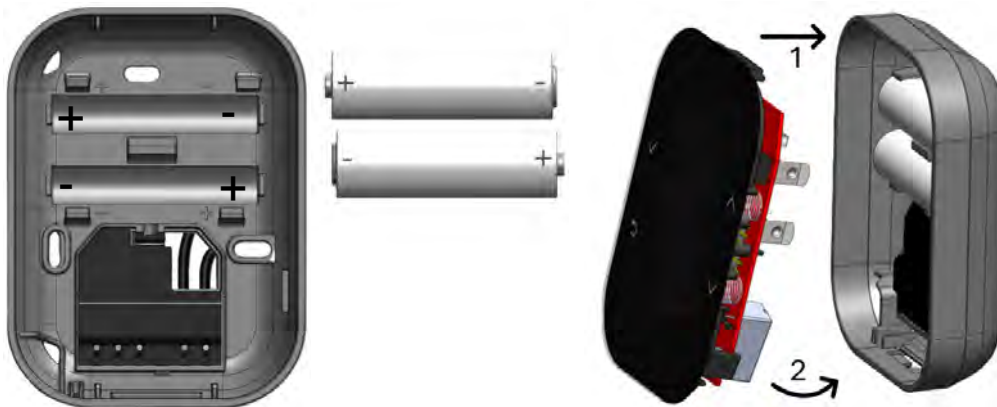
Figura 15 Chiusura Sensore ON/OFF
