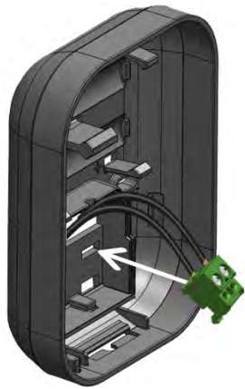
Figura 13 Riaggancio connettore Sensore ON/OFF
