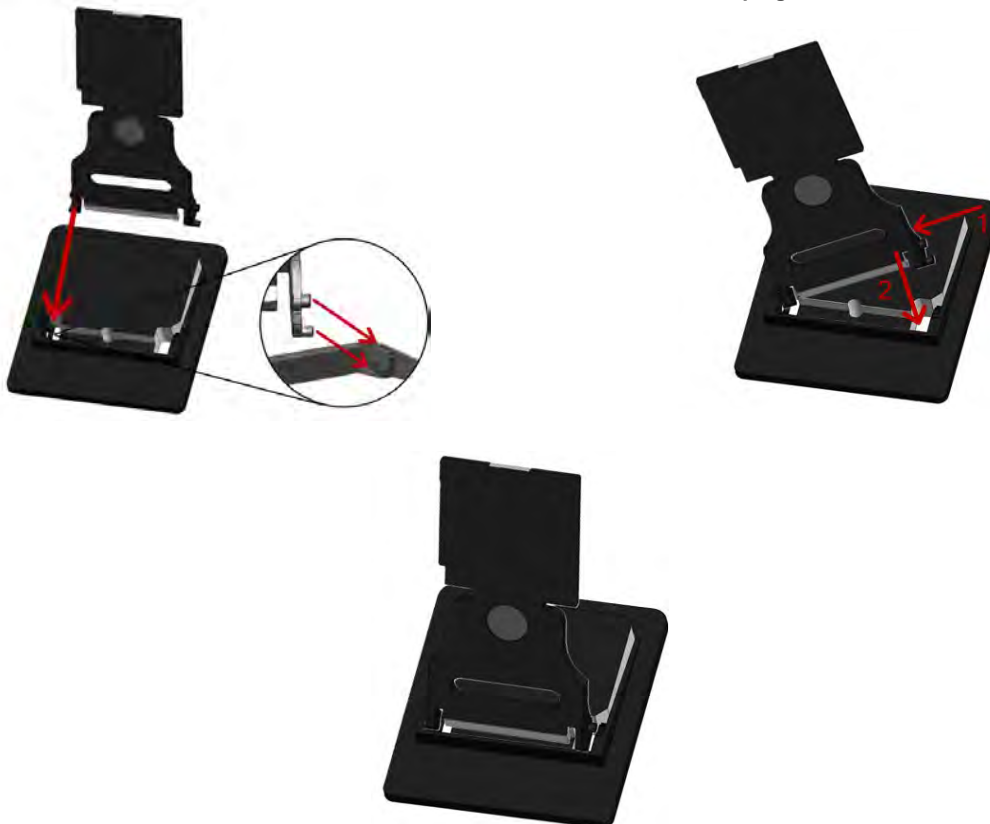
Figura 3 Assemblaggio parte superiore piedistallo
