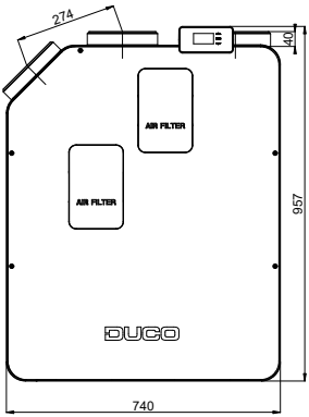
Vista frontale
