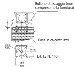
Dettaglio "A" tampone in gomma
