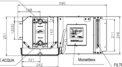
2-UNITÀ 2 TUBI
