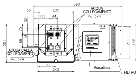
UNITÀ 4 TUBI
