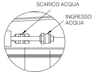
DETTAGLIO A
