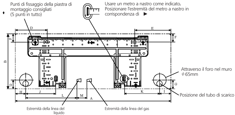
Piastra di montaggio ATXN25-35NV1B9
