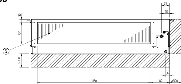
Vista A
