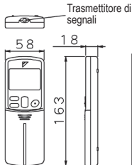
Telecomando a infrarossi (ARC433B70)
