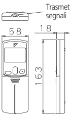
Telecomando a raggi infrarossi (ARC433A72)
