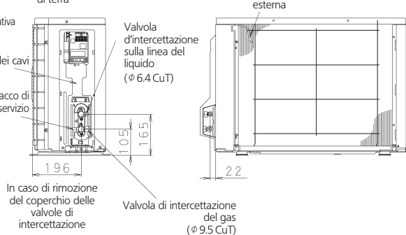
Morsetteria con collegamento di terra
