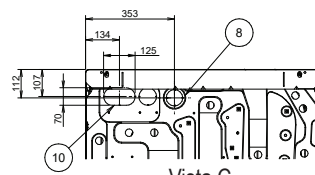
Vista C
