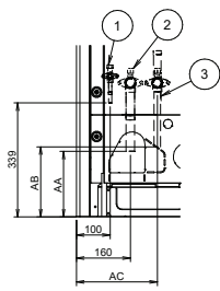
Dettaglio A
