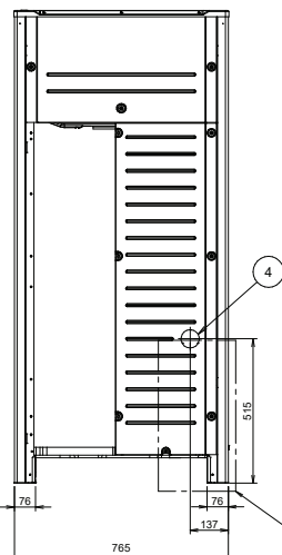
dettaglio B
