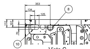
Vista C
