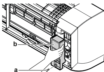
a Vite del coperchio di servizio b Coperchio di servizio
