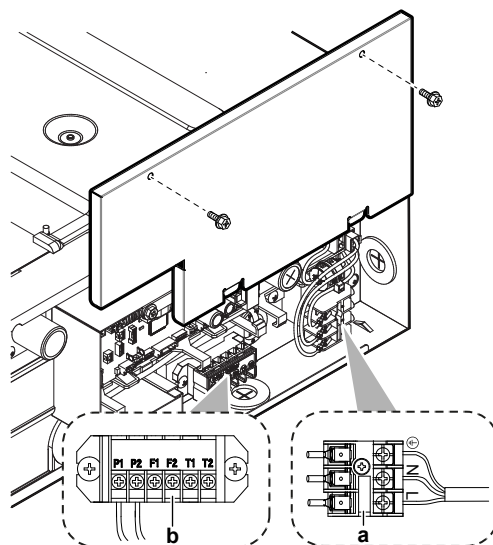
a Morsettiera di alimentazione b Morsettiera dell'interfaccia utente
