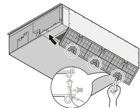
aspirazione inferiore
