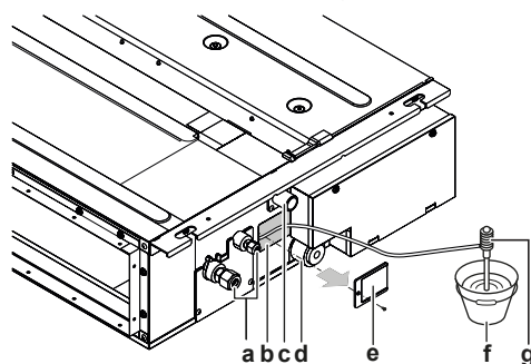
a Tubi del refrigerante b Ingresso dell'acqua c Collegamento di drenaggio d Uscita di drenaggio per la manutenzione e Coperchio dell'ingresso dell'acqua f Recipiente (aggiunta di acqua tramite l'ingresso dell'acqua) g Pompa portatile
