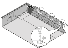
aspirazione posteriore
