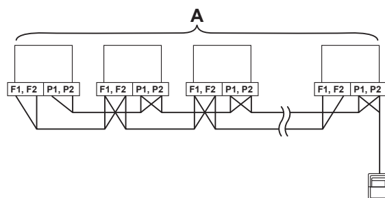
a Gruppo di comando a distanza (massimo 16 unità interne)
