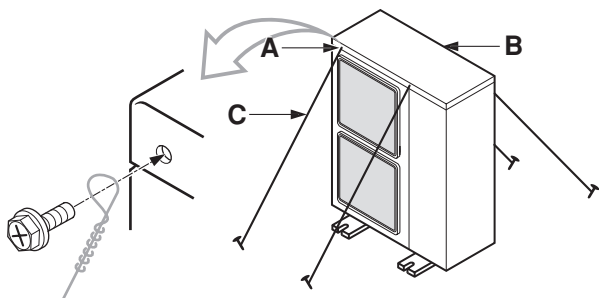
A Posizione delle due viti con cui fissare le funicelle alla parte frontale dell'apparecchio B Posizione delle due viti con cui fissare le funicelle alla parte posteriore dell'apparecchio C Cavi: non di serie
