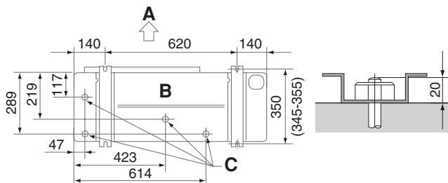
A Lato scarico B Vista dal basso (mm) C Foro di scarico
