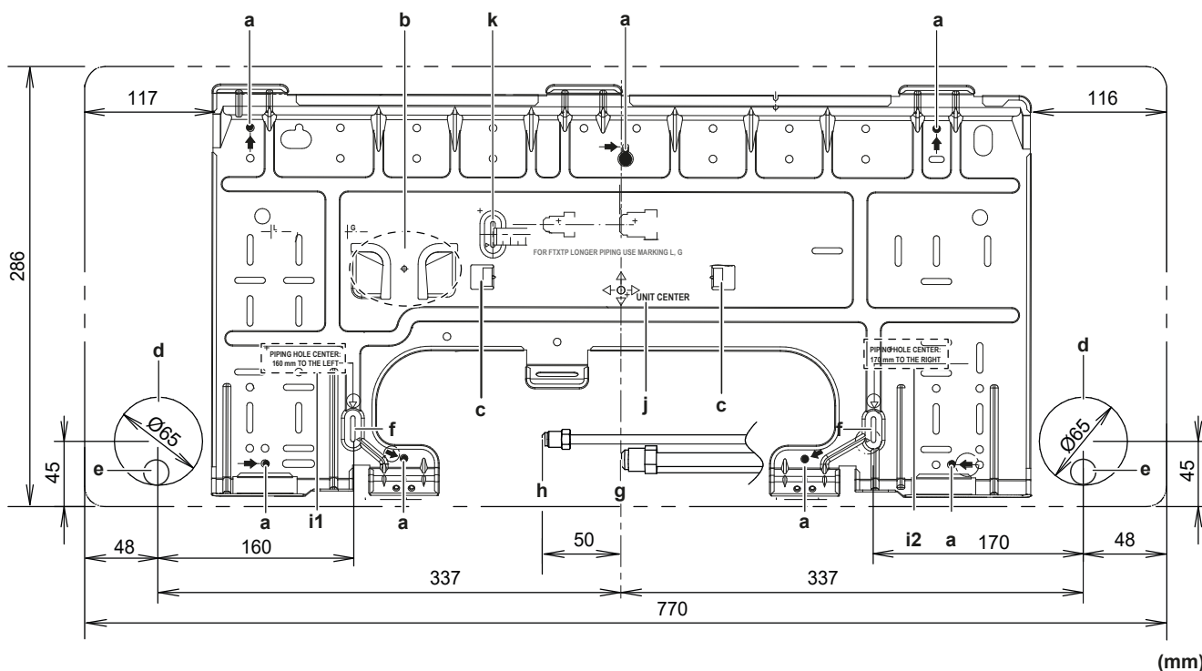
a Punti di fissaggio consigliati per la piastra di montaggio b Tasca per il coperchio della porta del tubo c Linguette per posizionare la livella d Foro passante nella parete Ø65 mm e Posizione del tubo flessibile di scarico f Posizione per il metro a nastro sul simbolo ">"
