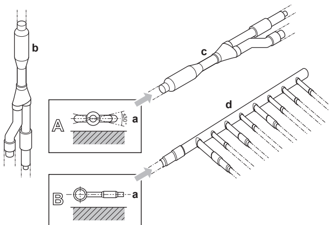
a Superficie orizzontale b Giunti Refnet montati verticalmente c Giunti Refnet montati orizzontalmente d Collettore
