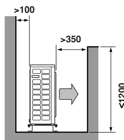
Vista laterale
