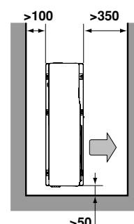
Vista dall'alto
