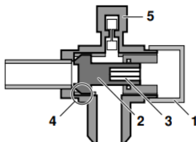
Figure 7- Caricamento dell'unità
