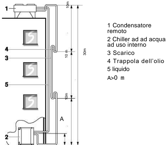
Figura 3-Collegamento del circuito refrigerante (1)
