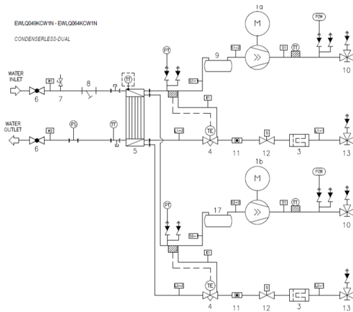
Figura 12- EWLQ 049 - 064 KCW1N Schema circuito refrigerante
