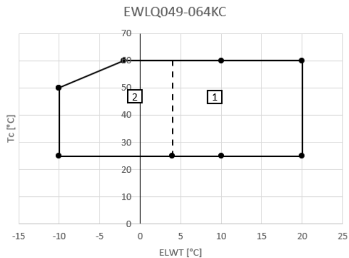
Figura 2-EWLQ049-064KC
