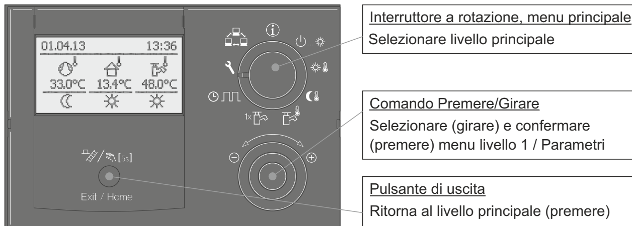
Immagine 2-1 Comandi – Unità di comando
